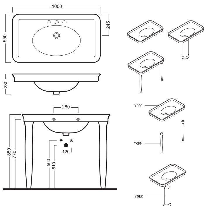
Схема установки раковины
