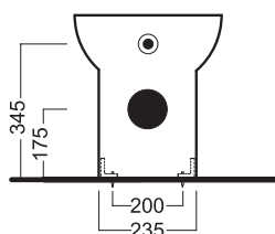
Схема установки унитаза
