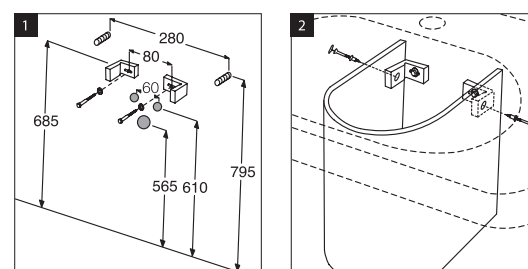
Схема установки раковины
