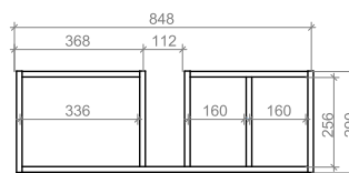
Вид сверху
