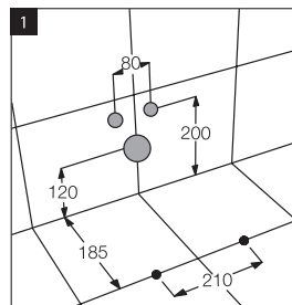
Схема установки биде
