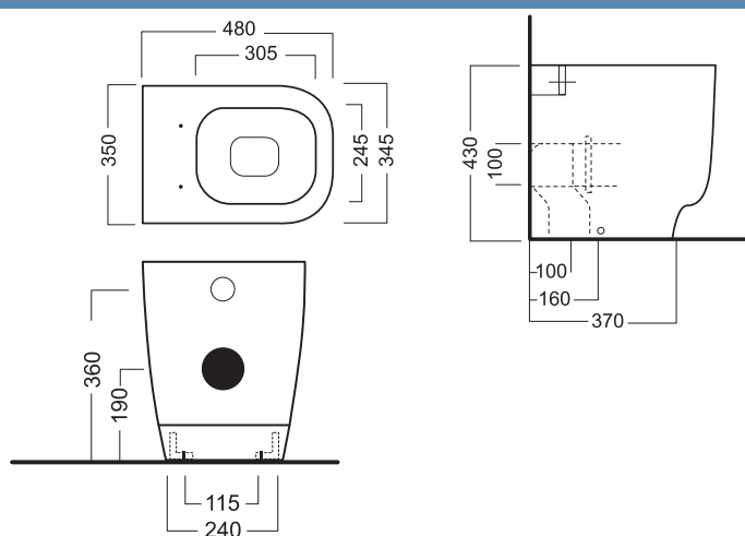
Схема установки унитаза
