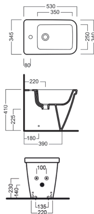
Схема установки биде
