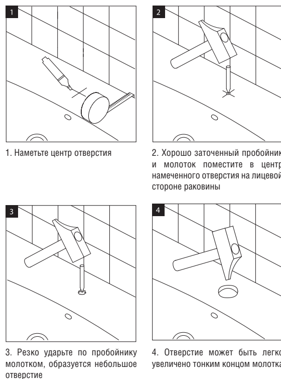
Как сделать отверстие под смеситель
