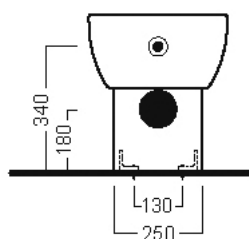
Схема установки унитаза
