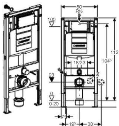
Монтажные размеры
