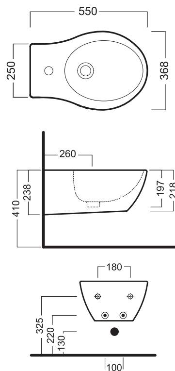
Схема установки биде
