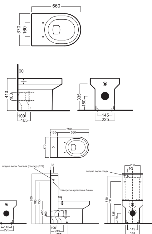
Схема установки унитаза
