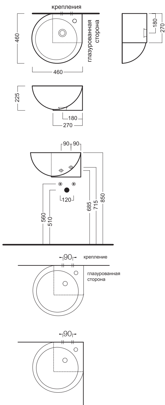
Варианты установки раковины
