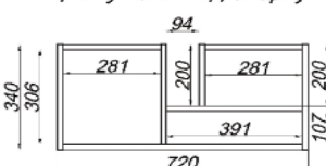
Ящик тумбы. Вид сверху
