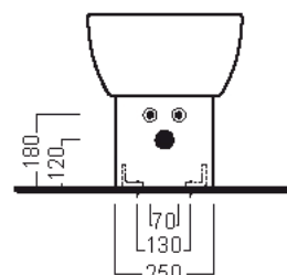
Схема установки биде
