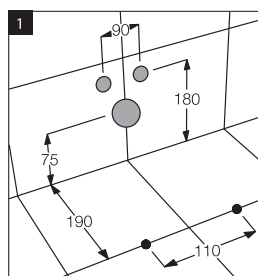
Схема установки биде
