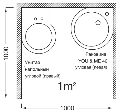
Установка угловых раковины и унитаза в туалетную комнату площадью 1 м 2
