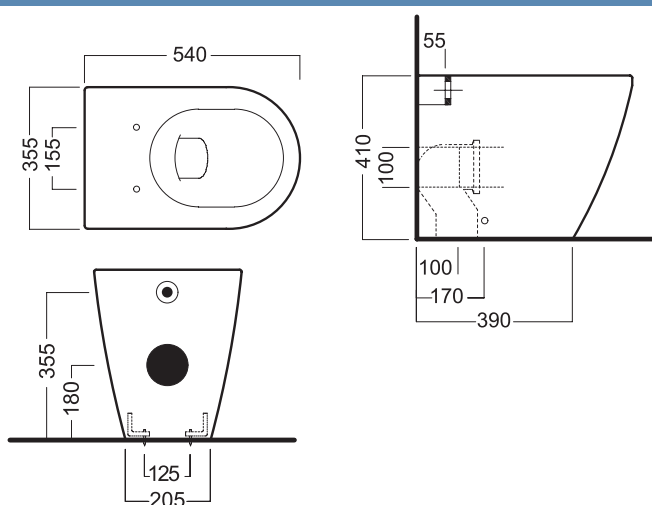
Схема установки унитаза
