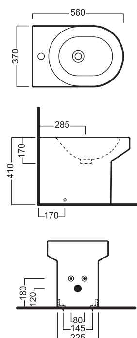
Схема установки биде
