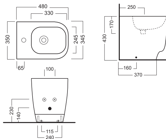
Схема установки биде
