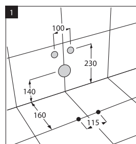
Схема установки биде
