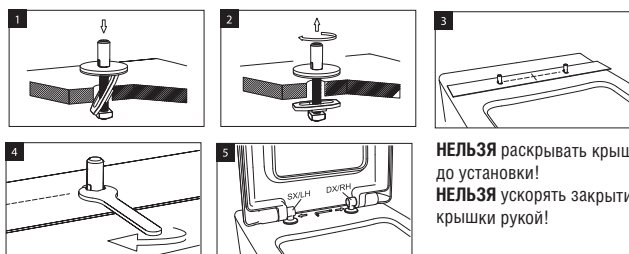
Схема установки сиденья
