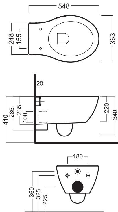
Схема установки унитаза
